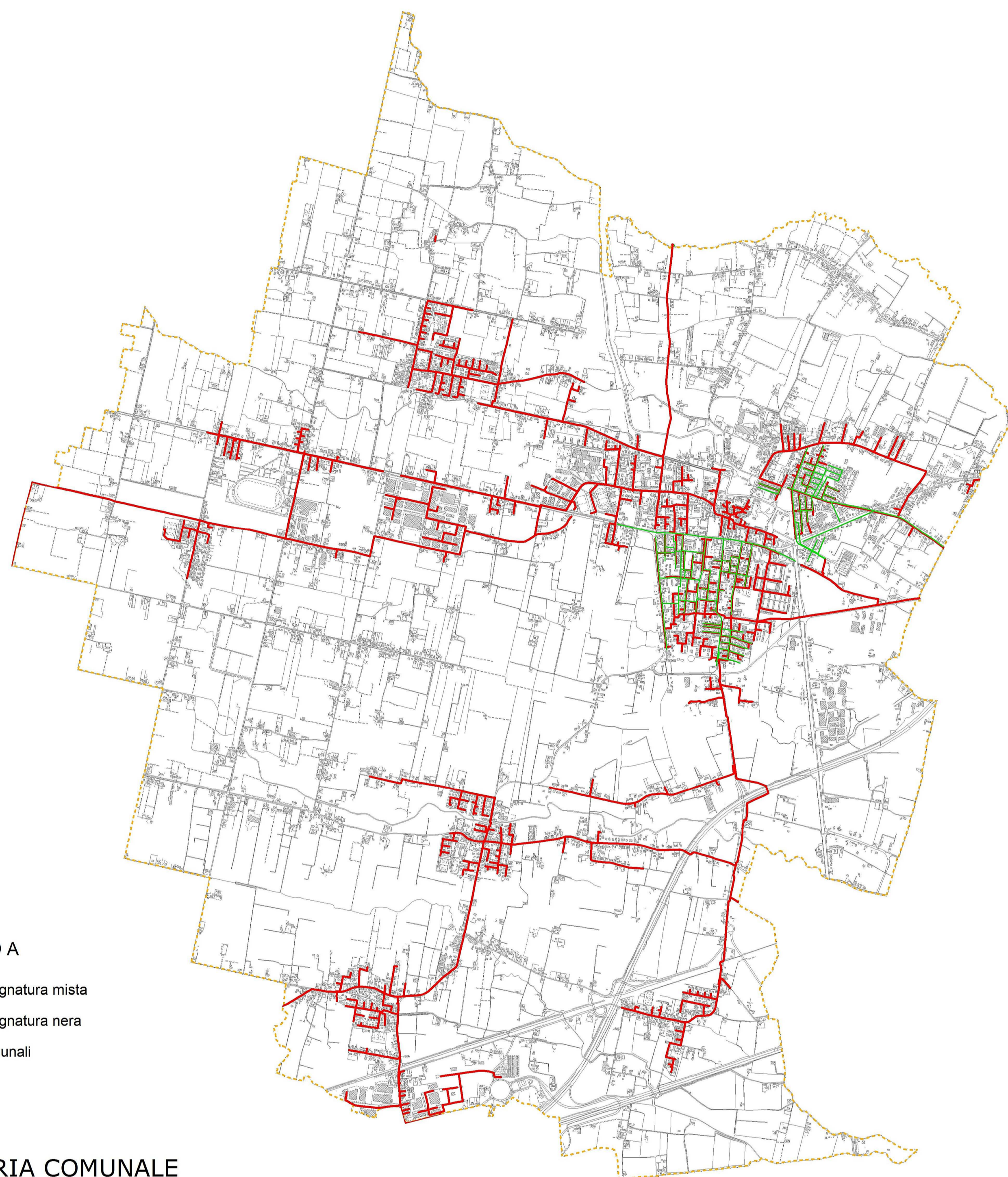
RETE FOGNARIA COMUNALE
